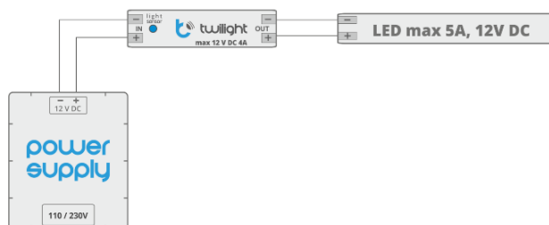
Rys. 1. – sposób podłączenia
