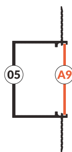
variant 05 - recessed 05-A9 spackle mounting variant 05 - wpustowy 05-A9 do szpachlowania
