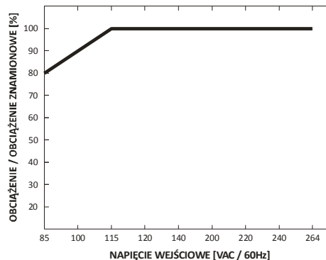
CHARAKTERYSTYKA OBCIĄŻALNOŚCI W ZALEŻNOŚCI OD NAPIĘCIA WEJŚCIOWEGO
